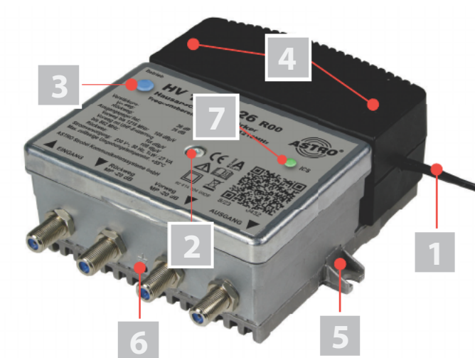
Bild 1: Verstärker HV 12K3626
