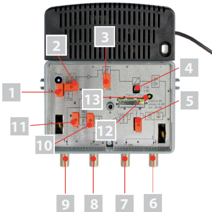
Bild 2: Verstärker HV 12K3626, Innenansicht
