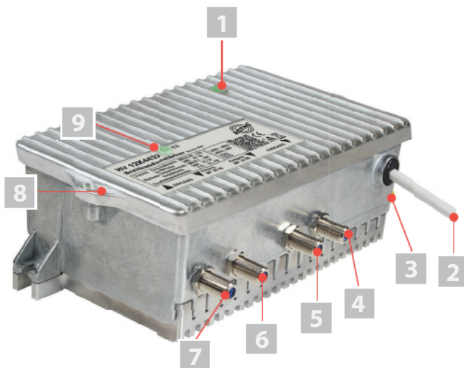
Bild 1: Verstärker HV 12K4432
