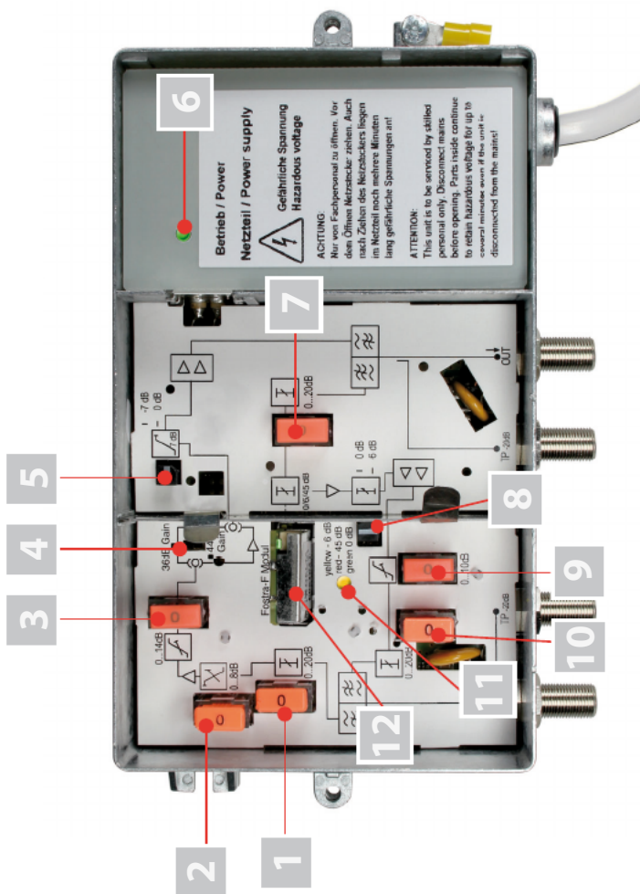
Bild 2: Verstärker HV 12K4432 Innenansicht; im Auslieferungszustand ohne Pads
